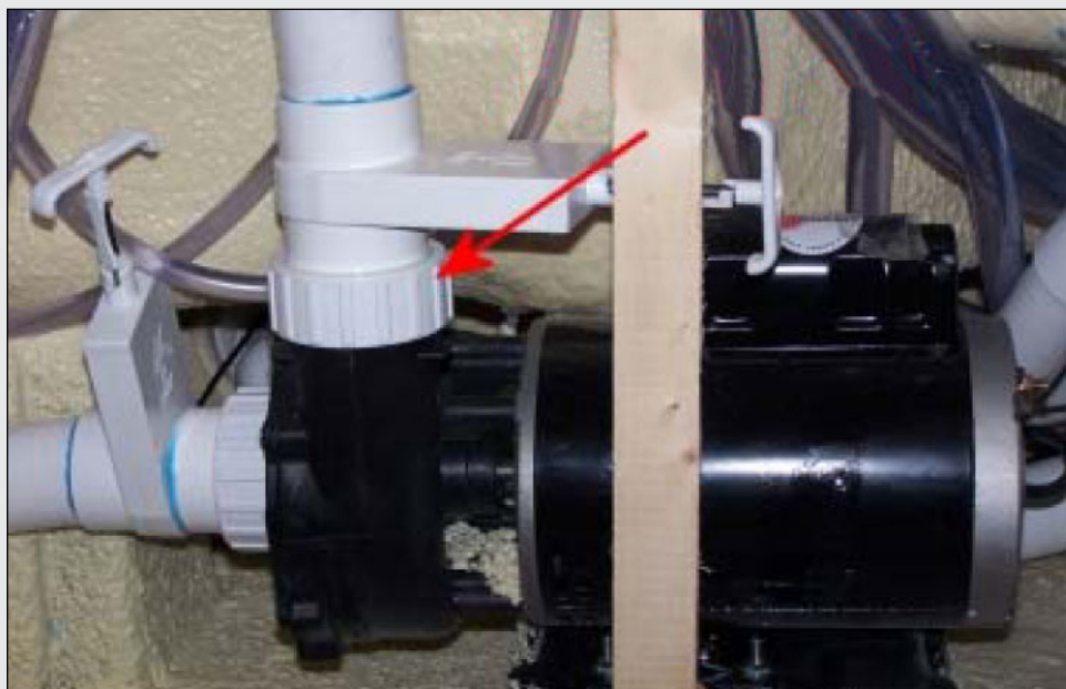
FIGURE 1.2 : BAGUE DE POMPE; DESERREZ POUR LAISSER S'ÉCHAPPER L'AIR
