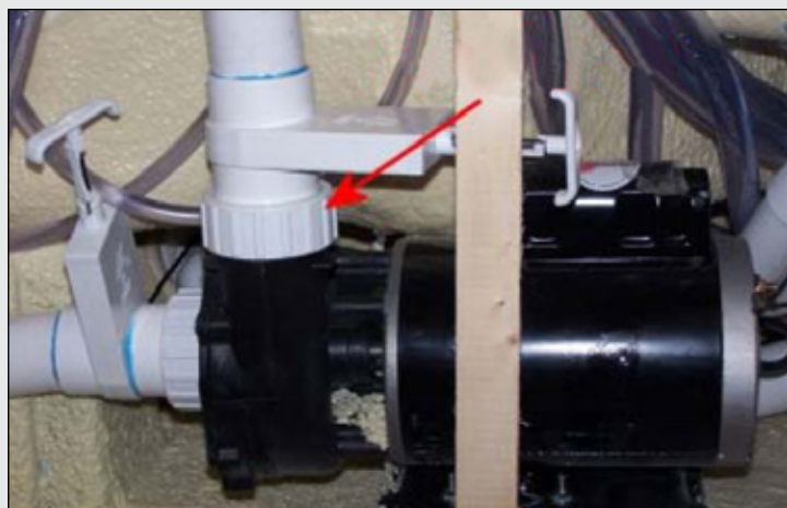
FIGURE 1.2b : BAGUE DE POMPE; DESERREZ POUR LAISSER S'ÉCHAPPER L'AIR
